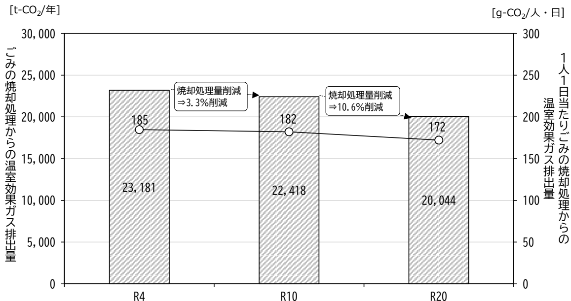
図 3-7 ごみの焼却処理からの温室効果ガス排出量の将来予測
