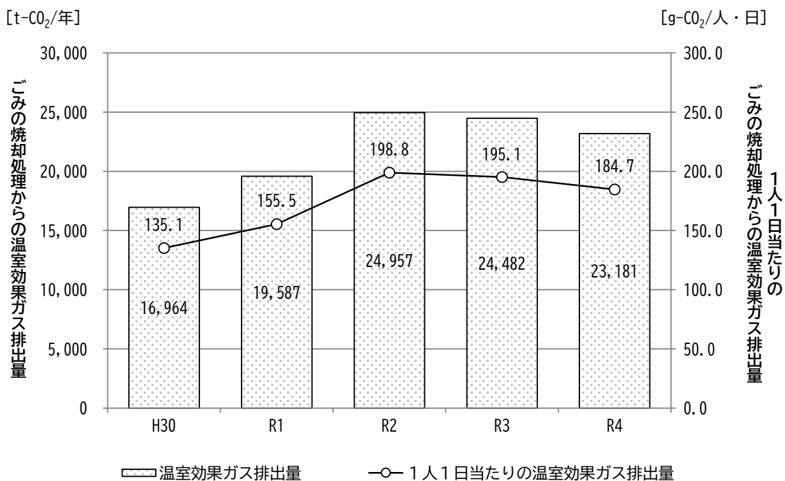
図 2-10 ごみの焼却処理からの温室効果ガス排出量の推移
