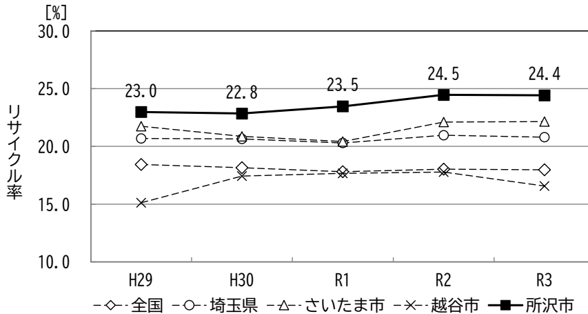
図 2-17 リサイクル率の比較
