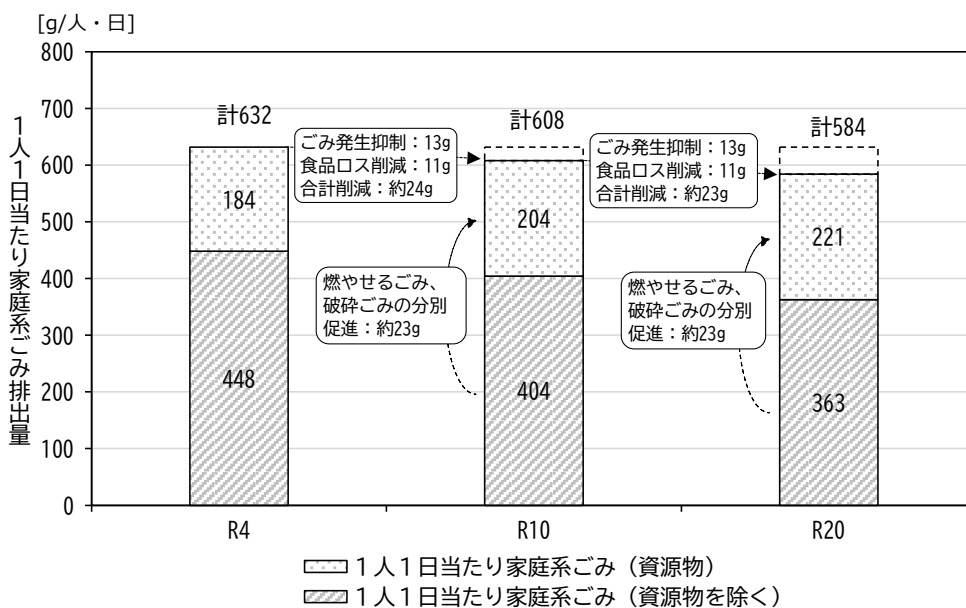
図 3-2 1人1日当たり家庭系ごみ排出量の将来予測
