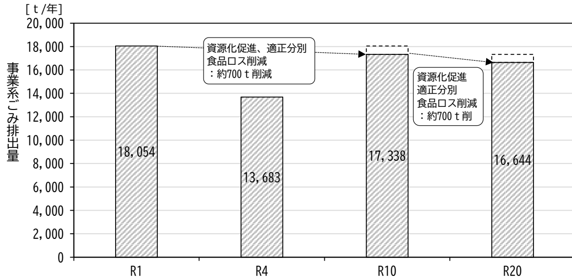
図 3-3 事業系ごみ排出量の将来予測
