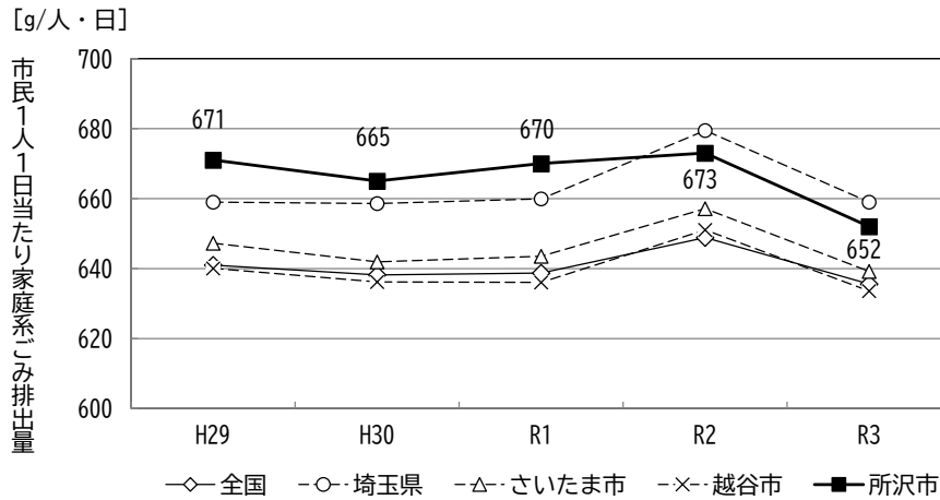
図 2-16 市民1人1日当たり家庭系ごみ排出量の比較
