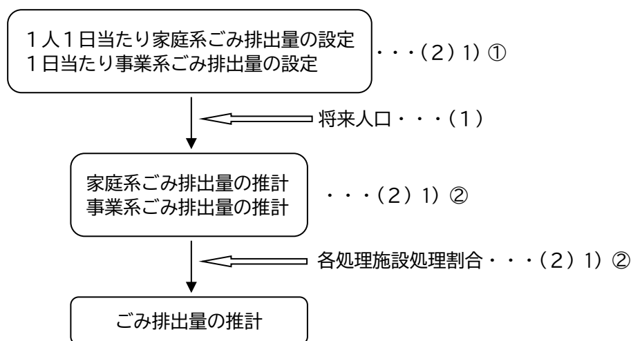
図資-16 将来ごみ量の推計方法
