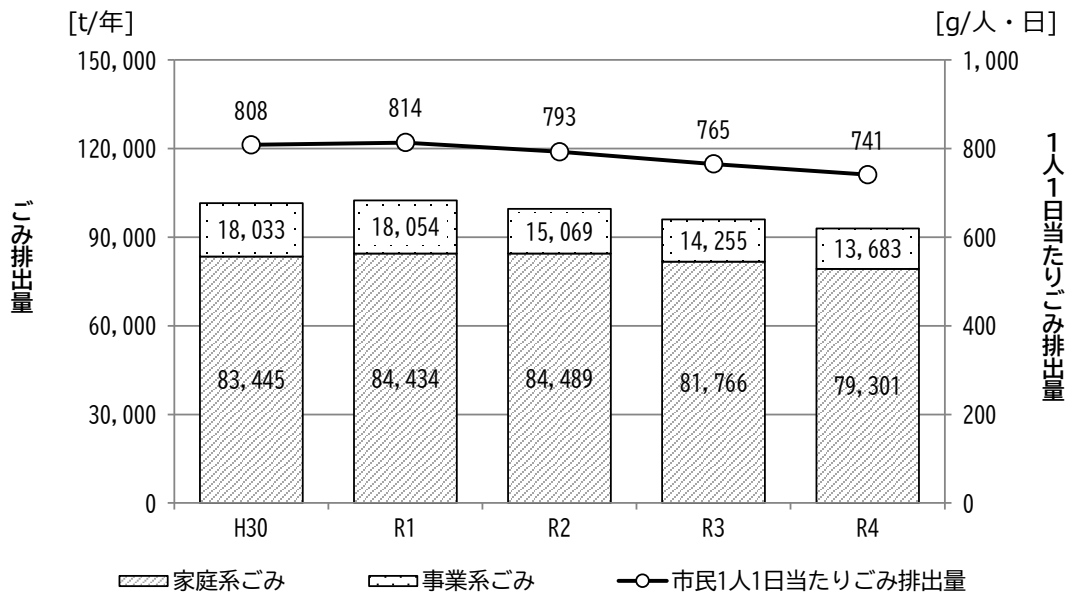
図 2-2 ごみの総排出量の推移
