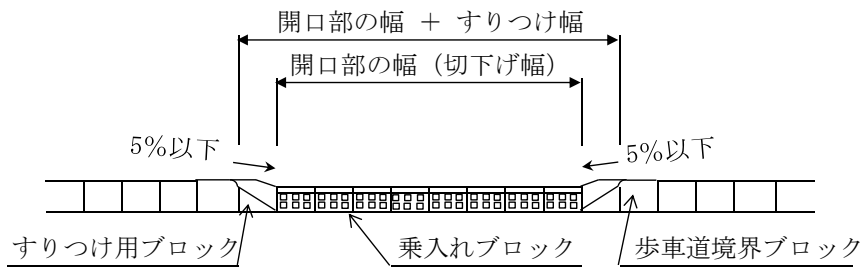
A-A' 断面図
