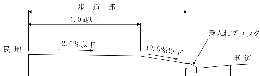
B-B' 断面図
